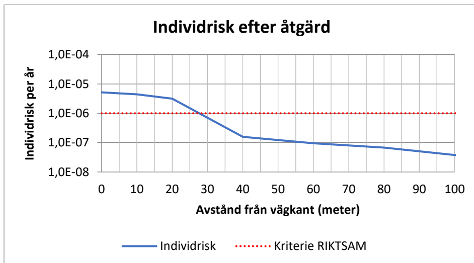
Figur 5.2. Individrisk vid planerad etablering vid åtgärd med brandklassad fasad.
