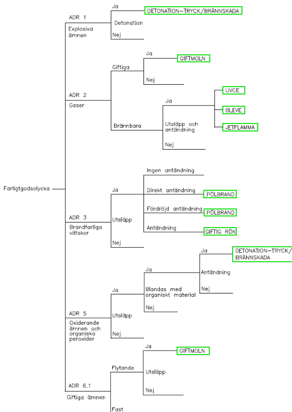
Figur 4.1. Möjliga konsekvensscenarier för väg 25/27 uppdelat utifrån identifierade ADR-klasser.
