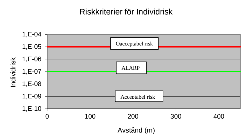
Figur 3.3. Illustration av kriterier för individrisk utifrån DNV:s kriterier.
