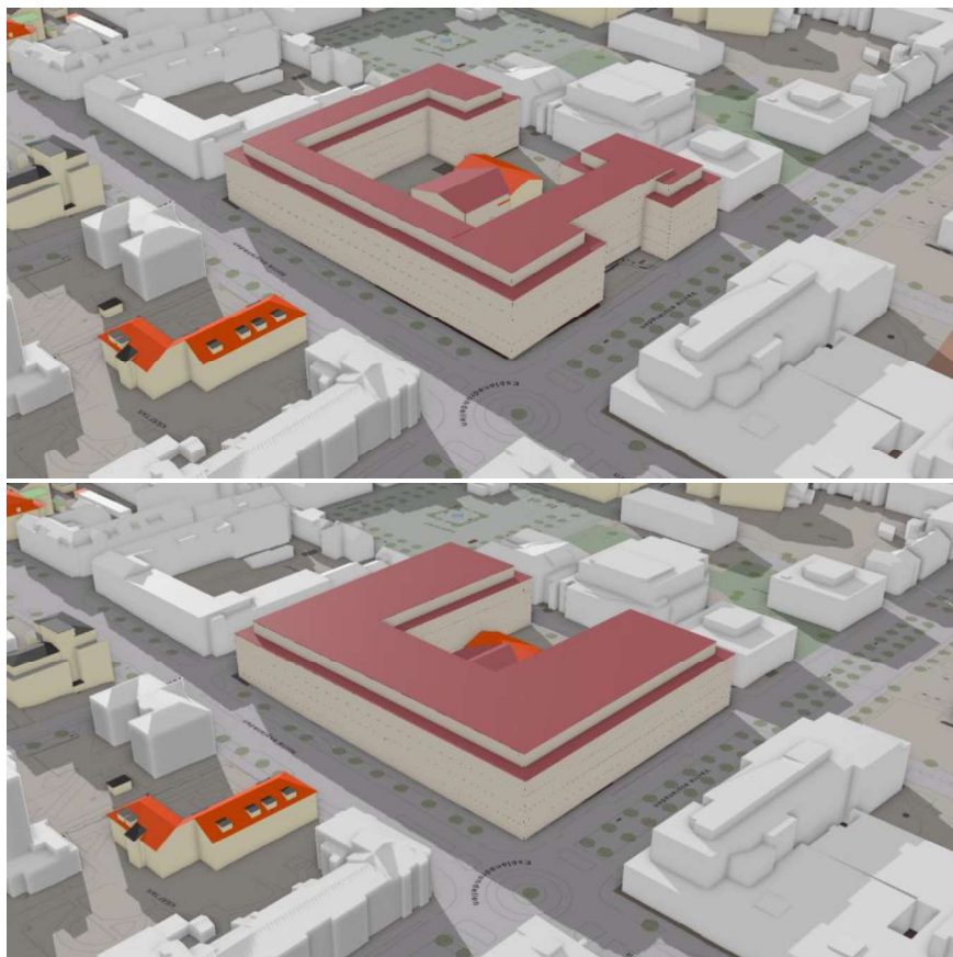
Bilderna ovan visar en 3D-modell över byggrätten sett från nordväst. Den övre bilden visar byggrättens hela utbredning höjd- och ytmässigt. Den nedre bilden visar en exempelbyggnation baserad på högsta höjder och högsta utnyttjandegrad.
